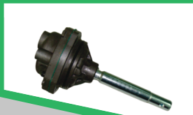
CILINDRO TRAVA DIFERENCIAL SCANIA SÉRIE 4 / 5 / NTG 2636262 / 2242842
